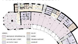
PŮDORYS HLAVNÍ BUDOVY
